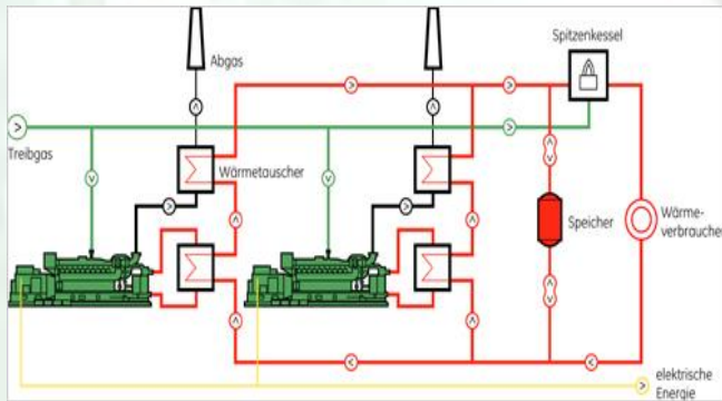
Typisches Fließbild einer Anlage
